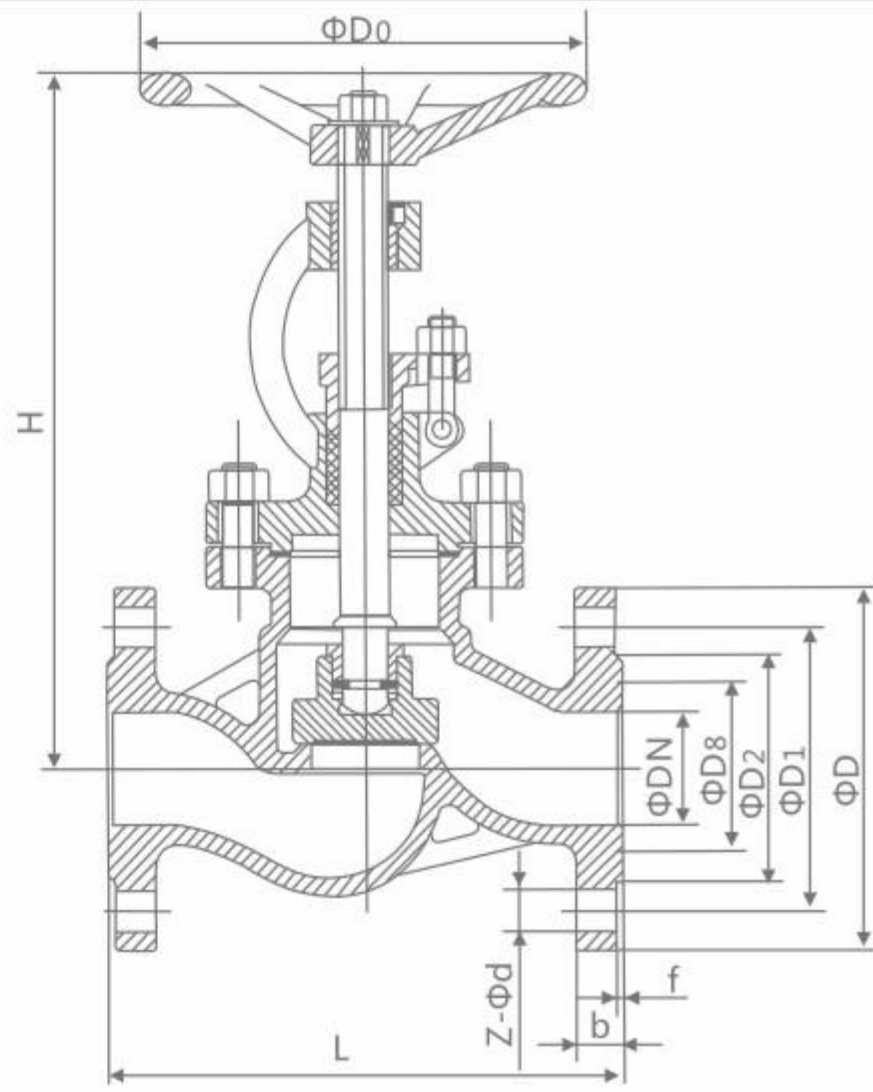
PN63 主要外形尺寸及连接尺寸 Main external and connection dimension
