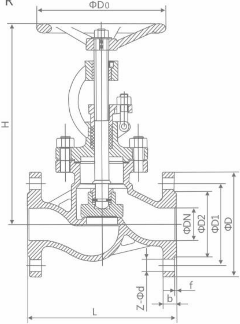
PN16 主要外形尺寸及连接尺寸 Main external and connection dimension
