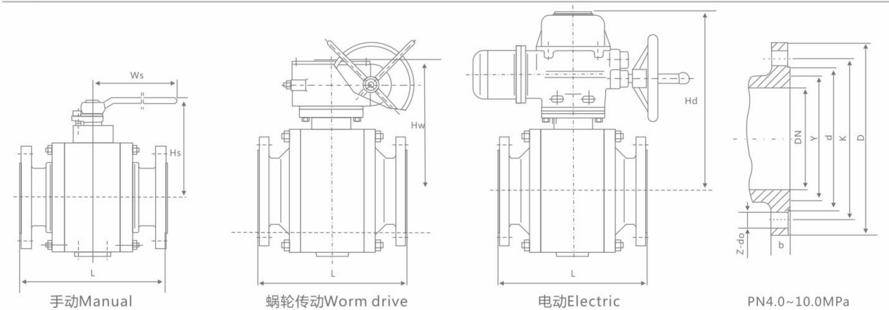
PN10 主要连接尺寸 Main connection dimensions
