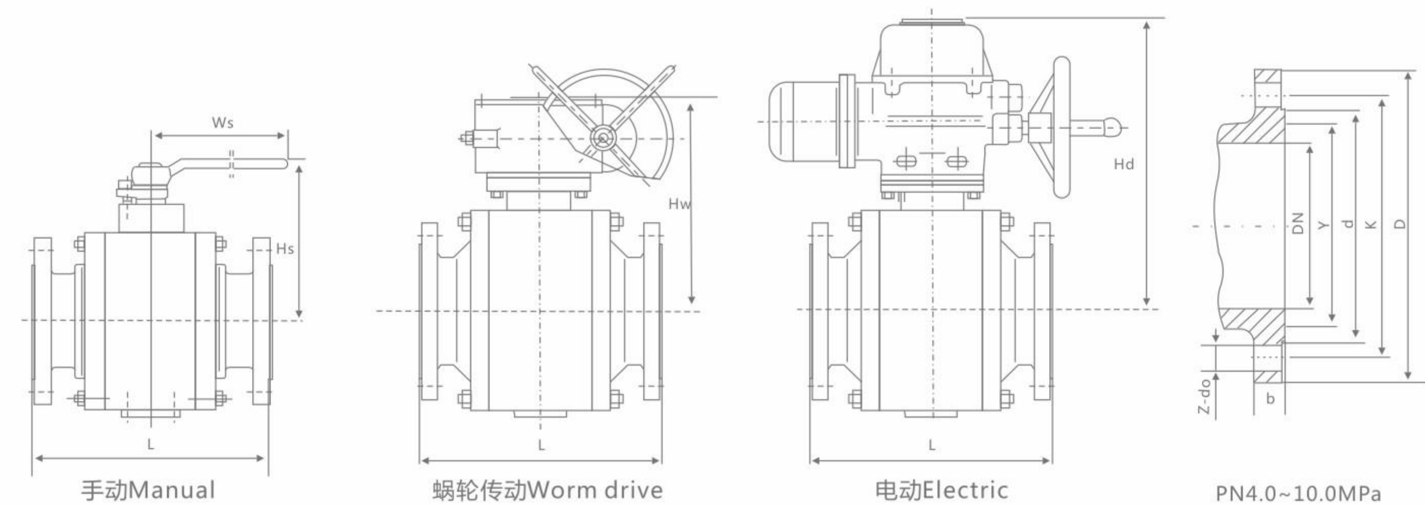
PN16 主要连接尺寸 Main connection dimensions
