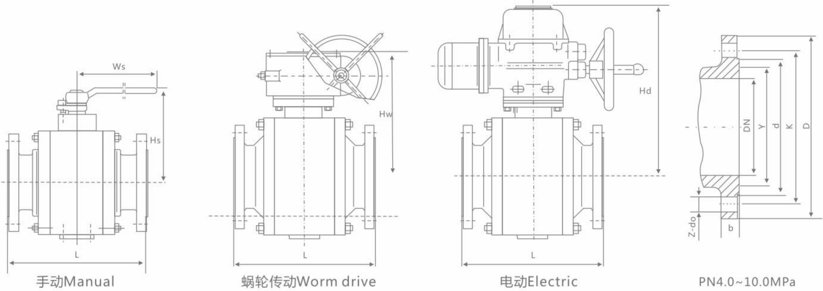
PN40 主要连接尺寸 Main connection dimensions
